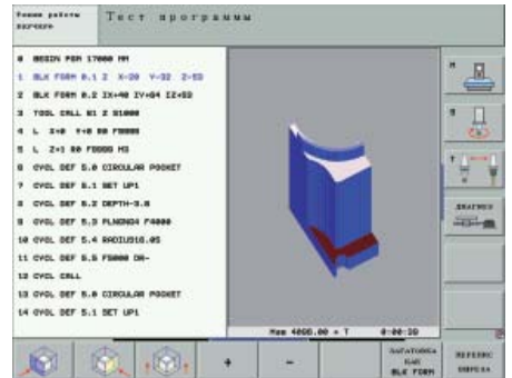
Тестирование программы
